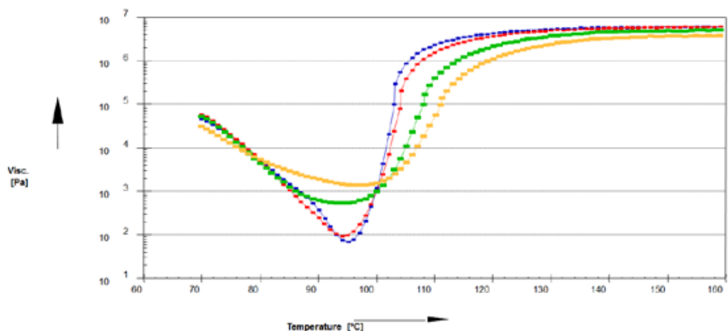
Viskositäts-[Pa] Temperatur [°C]- Diagramm:
